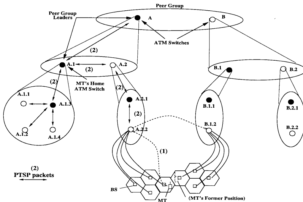
Fig. 27. Extended mobile PNNI.
